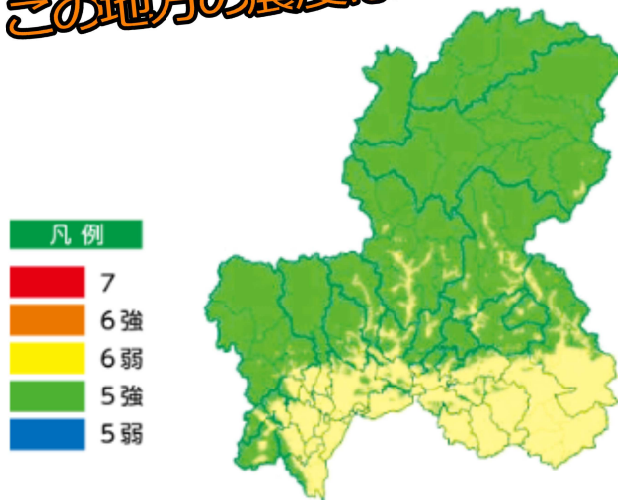
南海トラフ地震の想定震度分布図
